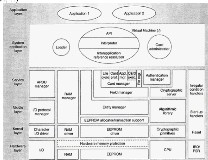
Structure d'un système d'exploitation de secure element 48
