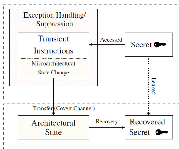
Attaque Covert Channel liées aux Micro Architectures
