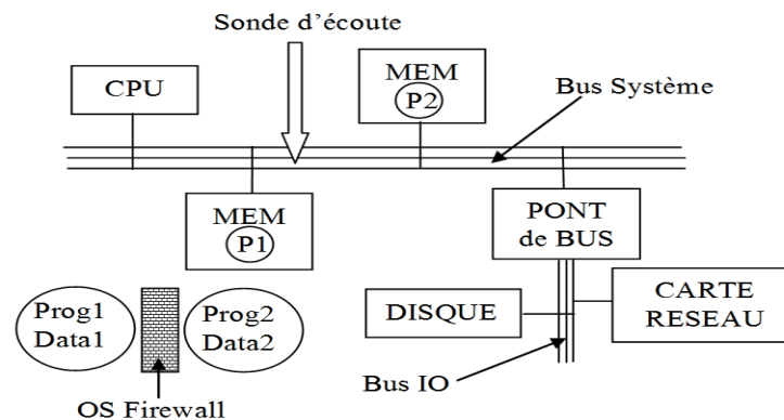
Le système PDP 11, 1970
