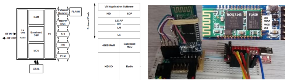
SoC CSR BC417143 (à gauche) et dispositif de chargement du firmware (à droite)
